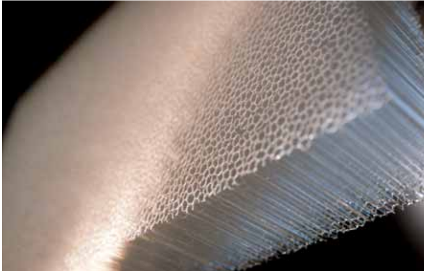
Wärmedämmend und lichtdurchlässig: Die Dämmschicht mit Kapillarstruktur.
