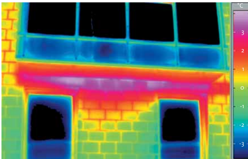
Die Thermografie-Aufnahme zeigt: Hier entweicht Wärme.
