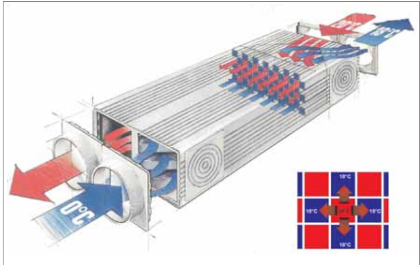
Der Kanalwärmetauscher enthält Warm- und Kaltluftkanäle im »Schachbrettmuster«: Die zunächst 0 °C kalte Zuluft wird durch die warme Abluft auf 18 °C erwärmt.
