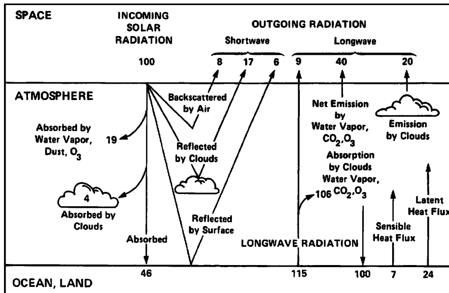
Abbildung 23: Ein schematisches Diagramm, welches die global gemittelten Anteile der Energiebilanz der Erde beschreiben soll. Diagramme dieser Art widersprechen der Physik .
